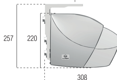
Installation au plafond
