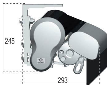
Installation au plafond
